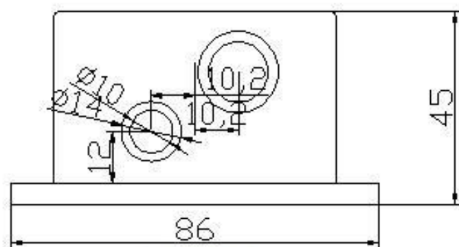
前视图
