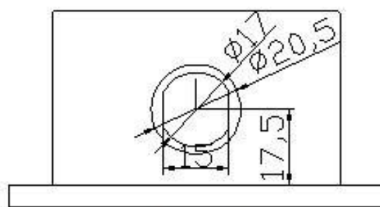
后视图
